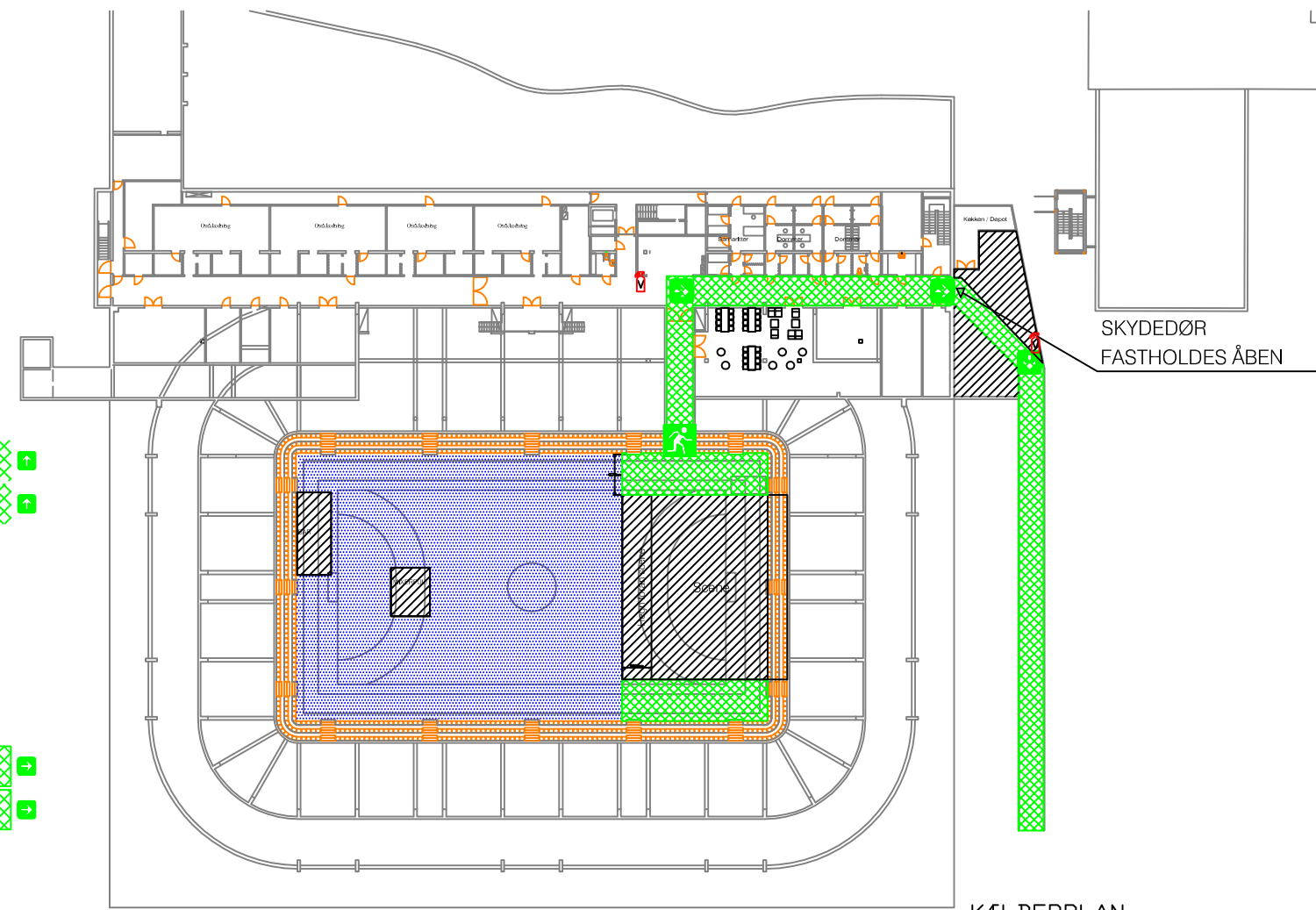
KÆLDERPLAN MÅL.1:300
